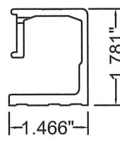
4 G-Channel 6063-T5
