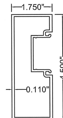
26 Jamb 6063-T6
