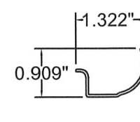
2 Sweep Clip 6063-T5
