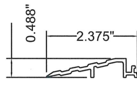
5 Leadup 6063-T5
