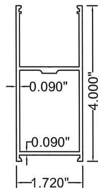
9 H4 6063-T5
