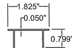
27 Jamb Snap 6063-T6
