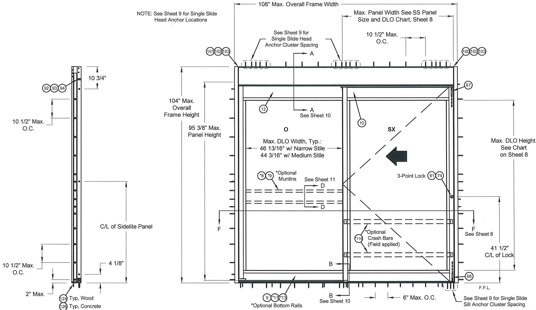
SIDELITE JAMB
